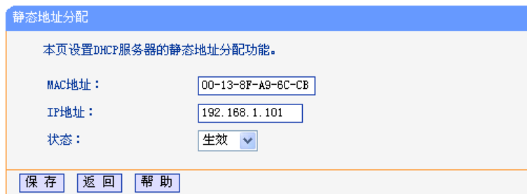
图 5-44 添加静态地址条目
