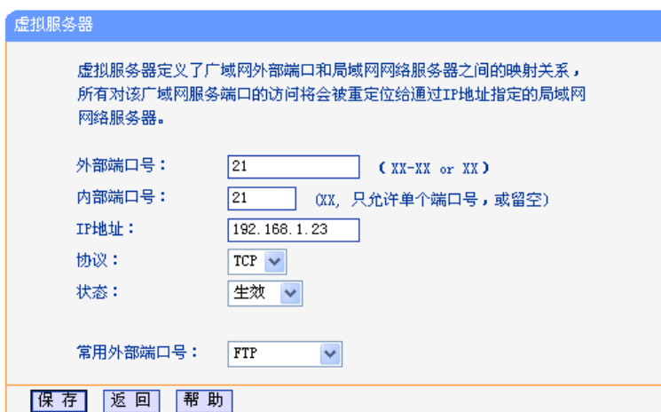
图 5-55 设置虚拟服务器条目
