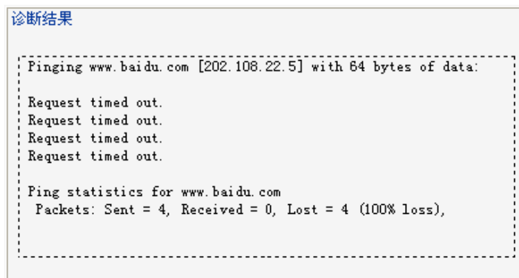
图 5-93 Ping 诊断结果—失败
