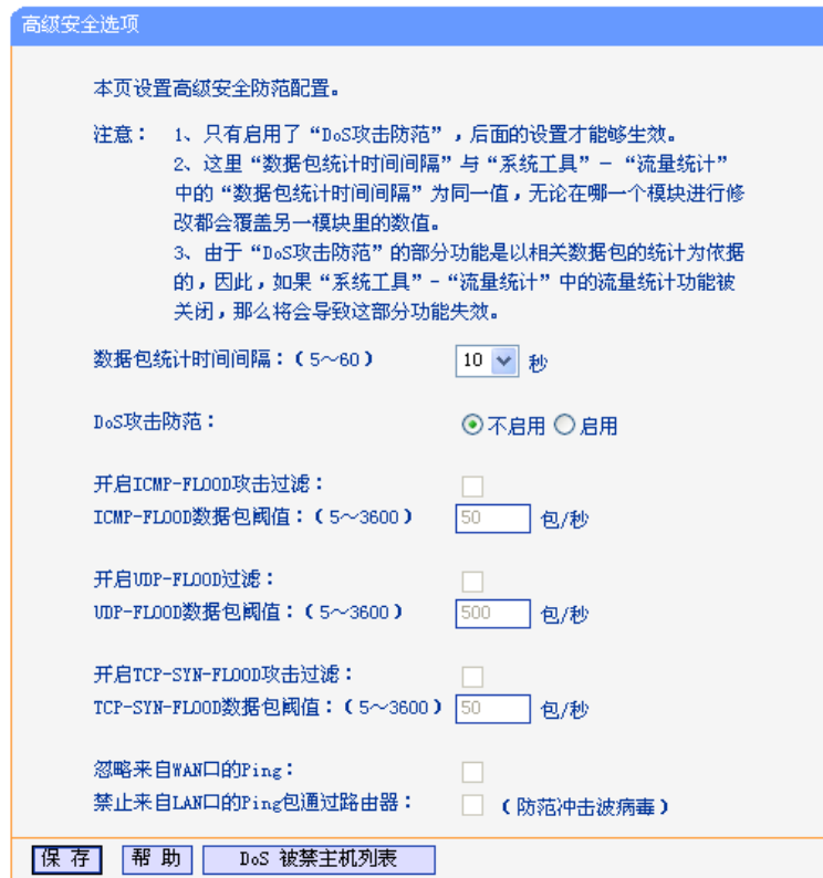
图 5-61 高级安全选项
