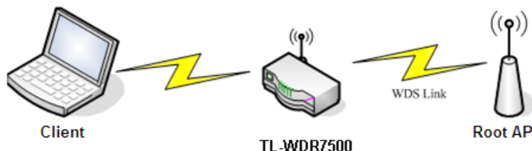
图 5-14 WDS 连接拓扑图
